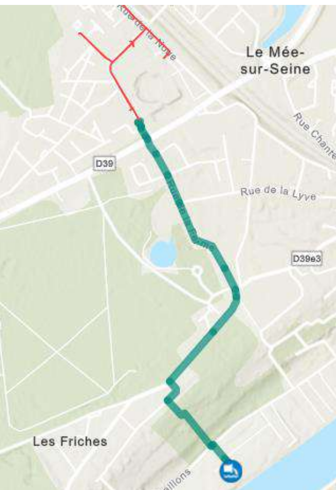
Exemple de tracé de raccordement (en vert) de la STEP (en bleu) au réseau existant (en rouge) par la voirie.
